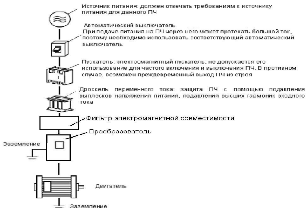
Схема электромонтажа основного силового контура
